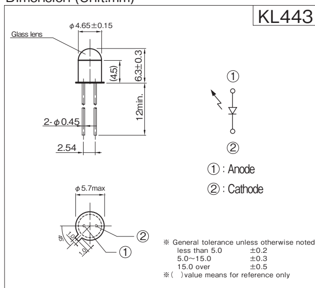
Dimension (Unit:mm)
