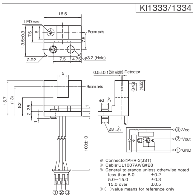
Dimension (Unit:mm)
