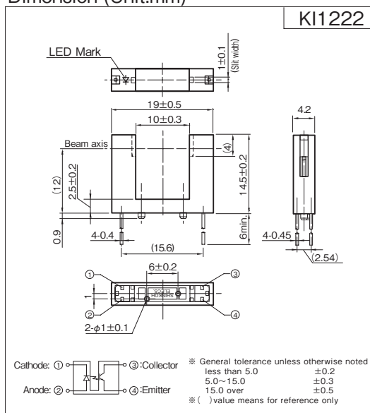
Dimension (Unit:mm)
