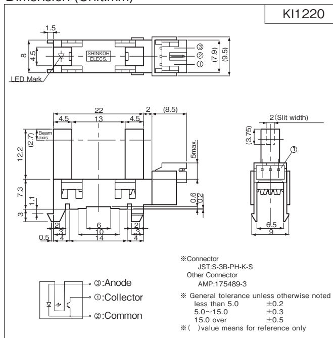
Dimension (Unit:mm)
