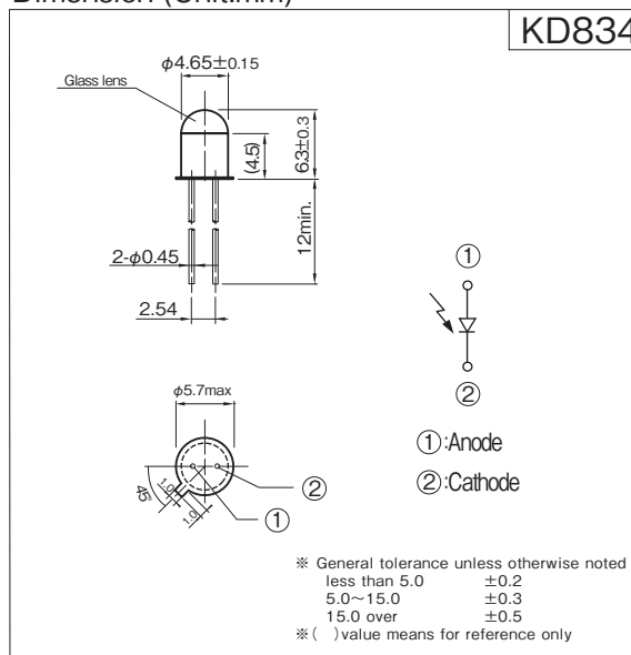
Dimension (Unit:mm)
